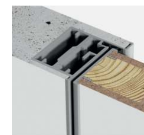
Монтаж коробки внешнее открывание
